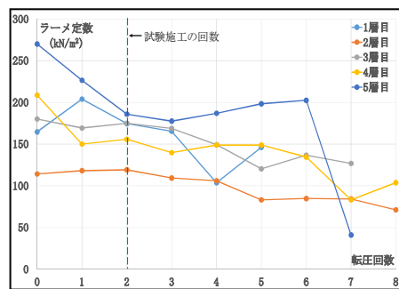
図-4 転圧回数による平均ラーメ定数
