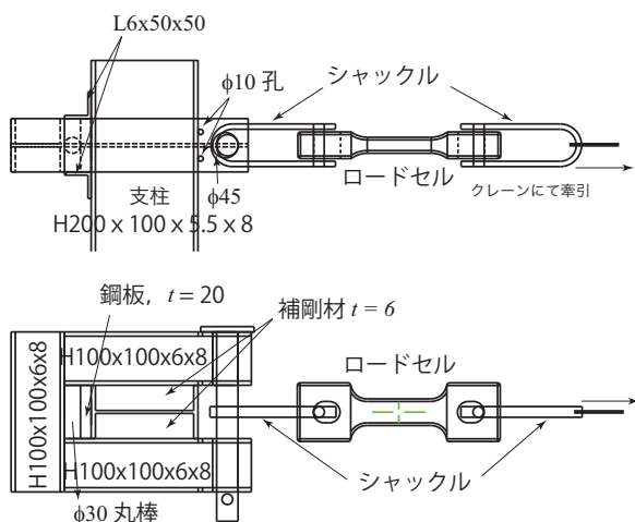
図－２ 載荷装置の概要
