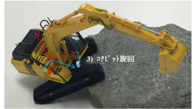
図-4 車体運動の分解
