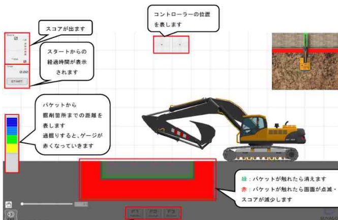
図-8 画面内容
