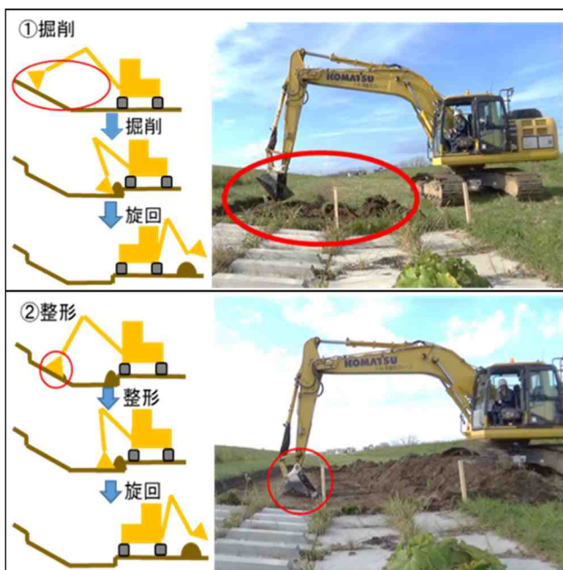
図-3 作業回数のカウント方法
