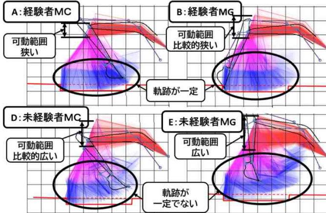
図-4 アーム挙動の比較
