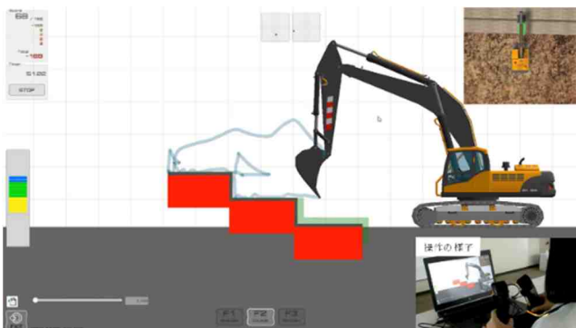
図-10 操作の軌跡
