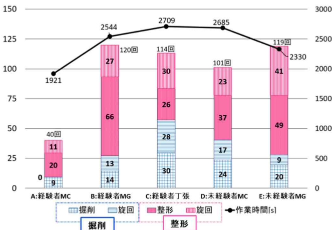
図-5 10m 当たりの作業回数・時間
